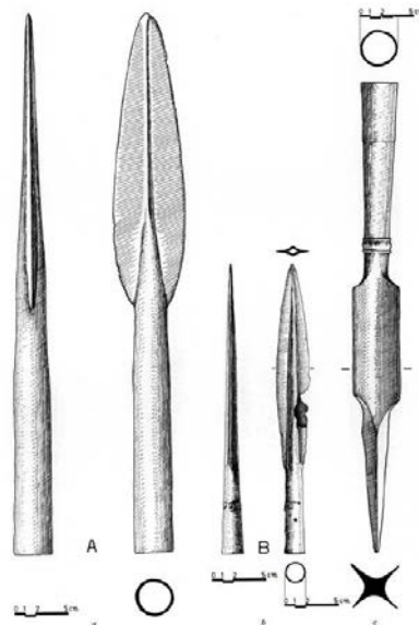
Fig. 9. — A. Pointe de lance A. (1 : 2) ; B. Pointe de lance B. (1 : 2) ; C. Talo de lance (1 : 3).
